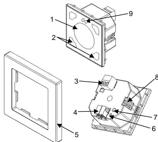
Рисунок 1: Flat 55 Display
