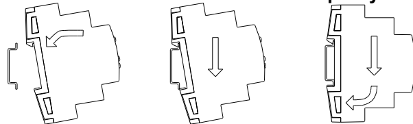
Рисунок 2. Монтаж и подключение ZPS640HIC230
