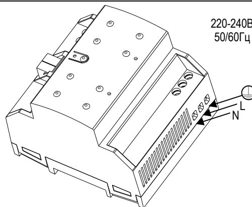
Рисунок 2. Монтаж и подключение ZPS640HIC230
