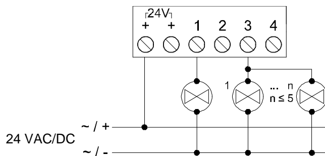
Σχήμα 2: Παράδειγμα καλωδίωσης: μια βαλβίδα ανά έξοδο και αρκετές βαλβίδες ανά έξοδο.
