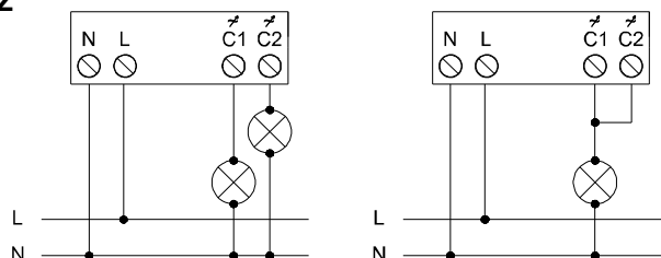
Σχήμα 2: Παραδείγματα καλωδίωσης (ανεξάρτητα κανάλια και σύνδεση κοινού καναλιού)
