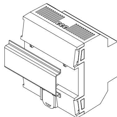
Σχήμα 3. Στερεώνοντας το DIMinBOX DX2 σε ράγα DIN
