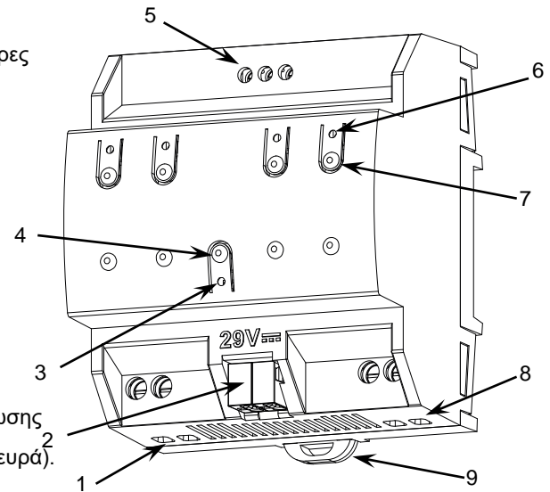
Σχήμα 1: DIMinBOX DX2
