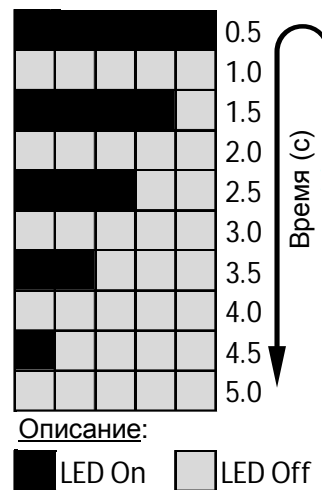
Рисунок 2. Уведомление об ошибке с помощью LED индикатора статуса канала DALI.
