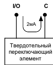
Выход управления на твердотельном элементе
