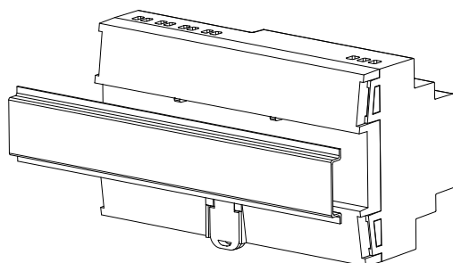
Σχήμα 3: Στερεώνοντας το ALLinBOX 88 σε ράγα DIN
