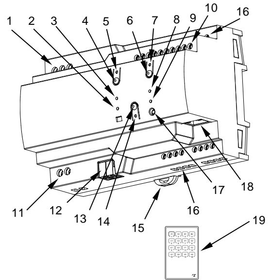
Σχήμα 1: ALLinBOX 88
