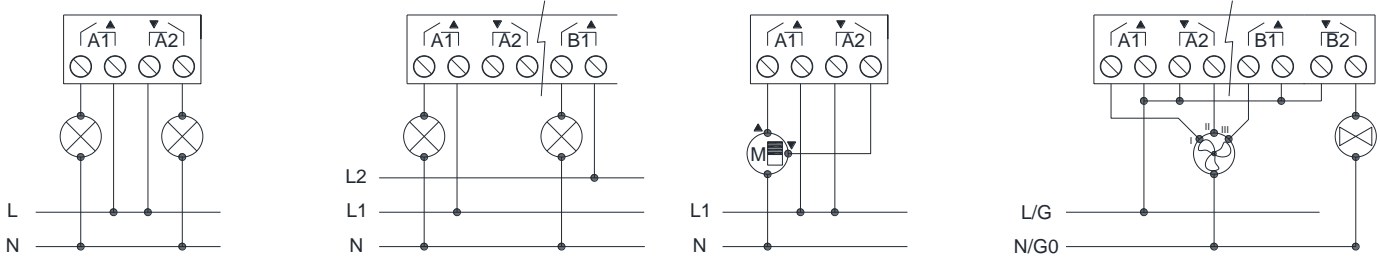
Σχήμα 1: Παραδείγματα συνδεσμολογίας (από πάνω προς τα κάτω και από αριστερά προς τα δεξιά): 2 φορτία, 2 φορτία συνδεδεμένα σε διαφορετικές φάσεις, κανάλι ρολού, ανεμιστήρας 3ων ταχυτήτων και βαλβίδες ανοικτό/κλειστό δισωλήνιου fan coil.
