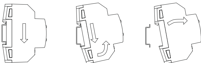
Figure 2. Montage du MINiBOX QUATRO sur rail DIN
