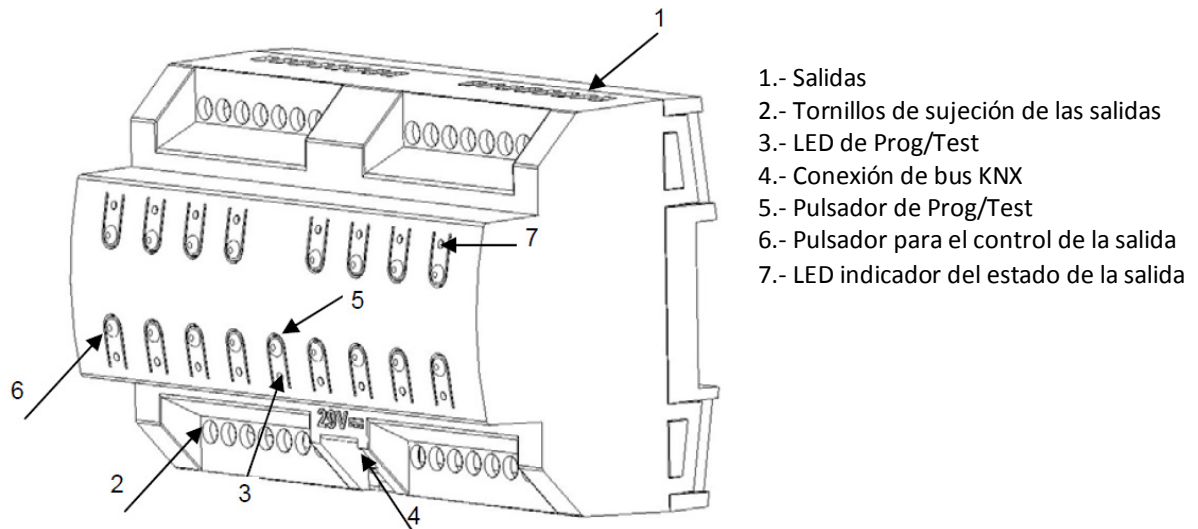
Figura 2. MAXinBOX 16. Esquema de elementos
