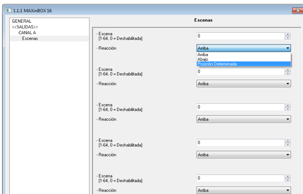
Figura 15. Escenas
