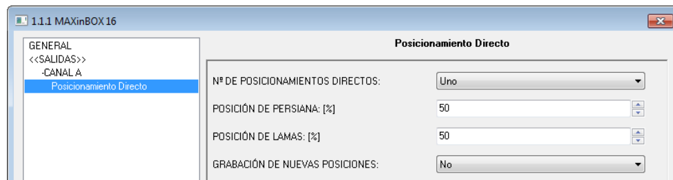
Figura 17. Posicionamiento directo
