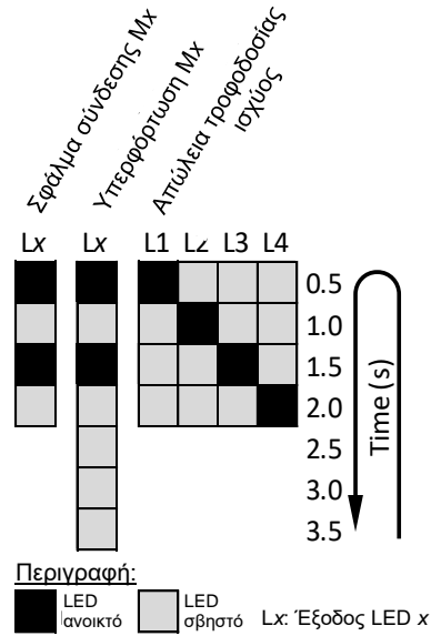
Σχήμα 2: Ειδοποίηση σφάλματος μέσω LED κατάστασης γρίλιας
