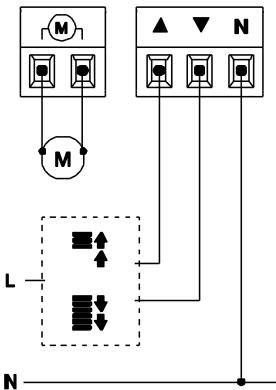
Σχήμα 2. καλωδίωση παράδειγμα
