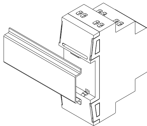
Σχήμα 3: Στερεώνοντας το MINiBOX QUATRO σε ράγα DIN
