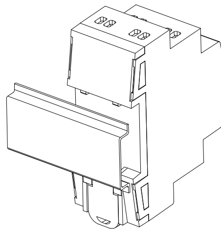
Figura 3: Montaje de MINiBOX 40 v2 en carril DIN
