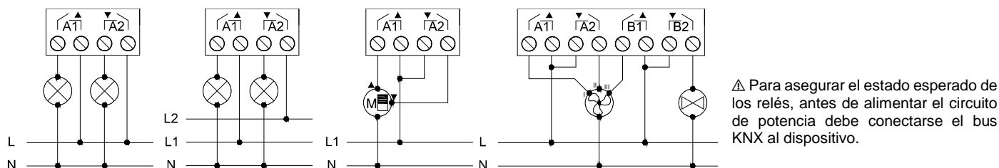
Figura 2: Ejemplo de conexionado (de izquierda a derecha): 2 cargas, 2 cargas a fases distintas, persiana y fan coil
