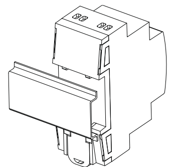
Figura 3: Montaje de MINiBOX 0-10V X2 en carril DIN
