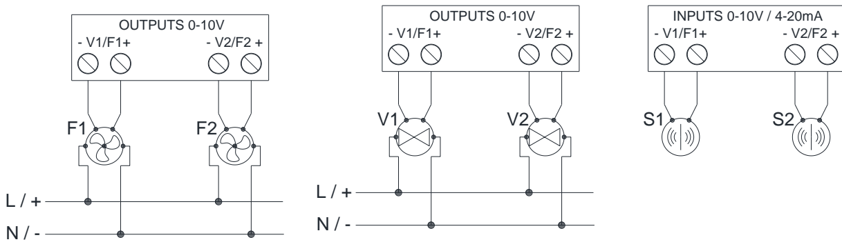
Figura 2: Ejemplos de conexionado
