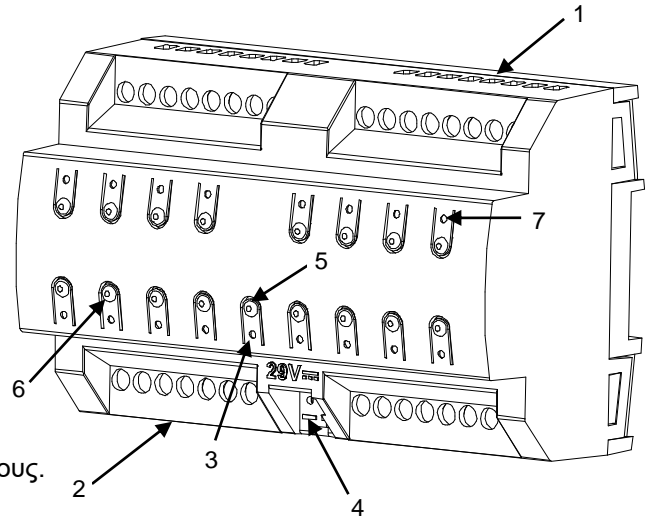
Σχήμα 1. MAXinBOX FANCOIL 4CH2P
