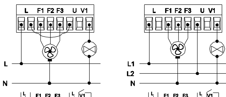
Σχήμα 2. Παραδείγματα καλωδίωσης FAN COIL με την ίδια και με διαφορετικές φάσεις
