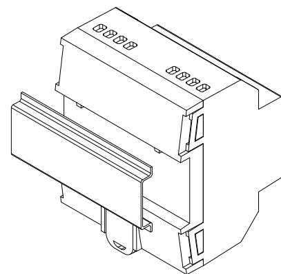
Σχήμα 3: Στερεώνοντας το MAXinBOX FANCOIL 2CH2P v2 σε ράγα DIN
