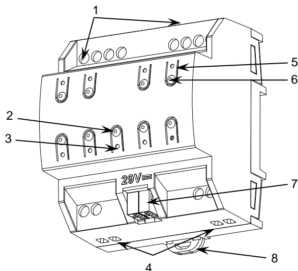
Σχήμα 1: MAXinBOX FANCOIL 2CH2P v2
