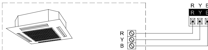
Σχήμα 2. Συνδέοντας το KLIC-LG1 στον εξοπλισμό Air Condition
