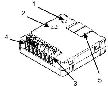
Σχήμα 1. KLIC-LG1
