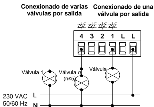
Figura 2: Ejemplo de conexionado: varias válvulas por salida y una válvula por salida
