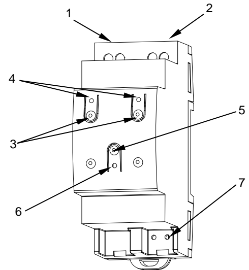
Σχήμα 1: FANinBOX 230V 1CH
