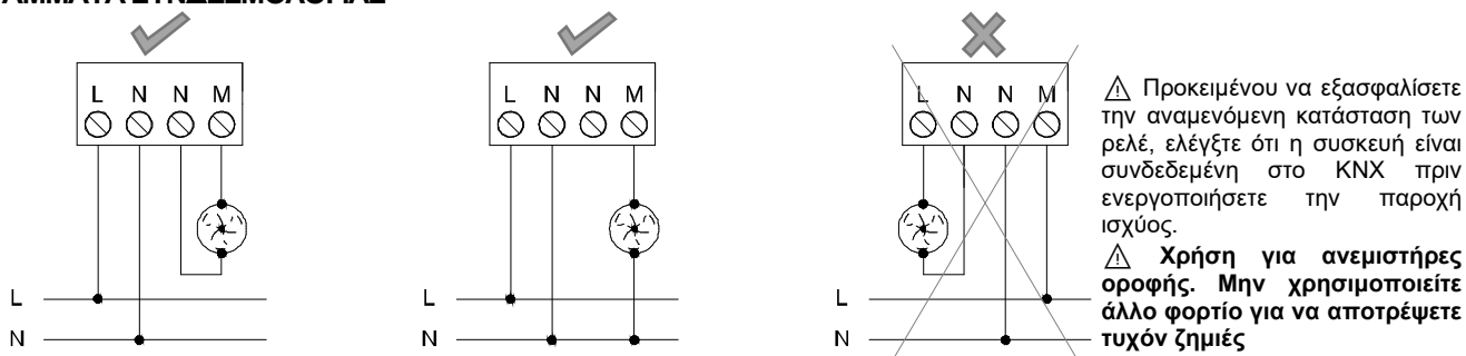
Σχήμα 2: Διάγραμμα συνδεσμολογίας ενός ανεμιστήρα
