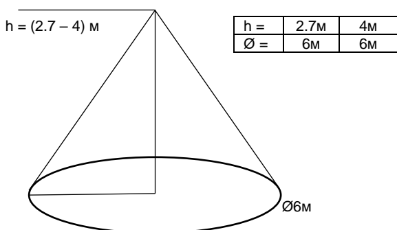
Рисунок 2: Дальность обнаружения движения
