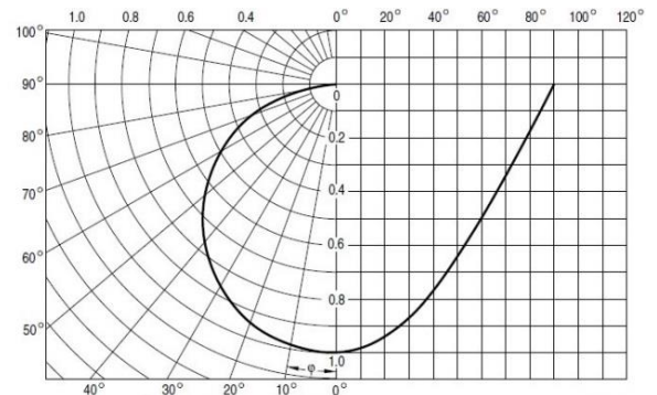
Figure 3: Sensibilité du capteur du niveau d'éclairage
